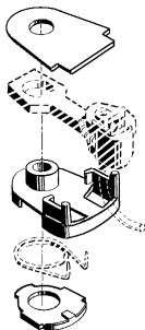
Draft Gear Box Lid
